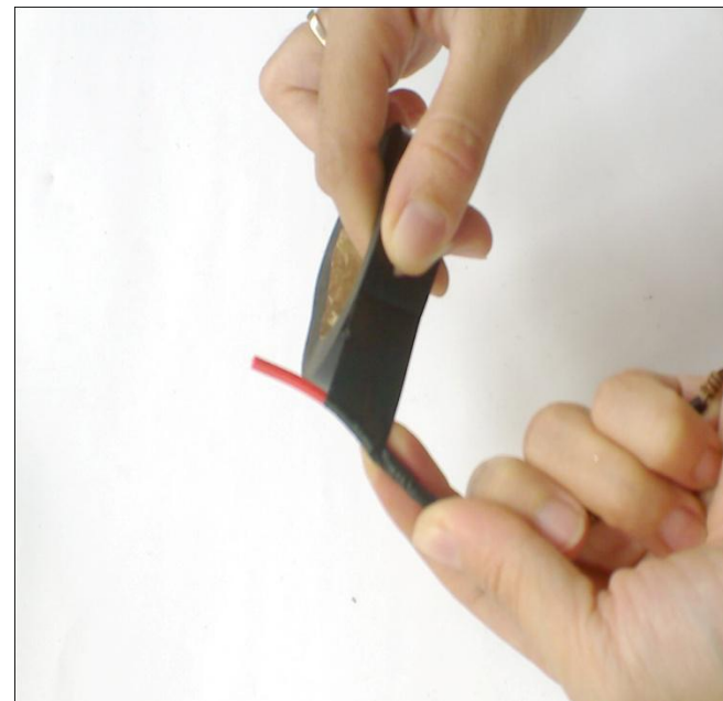
Bước 5 Cách điện mỗi nối
