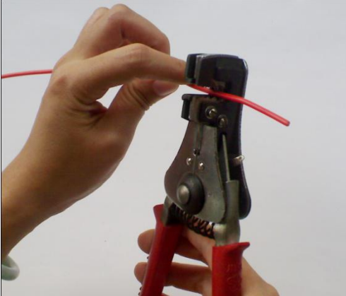
Bước 1 Bóc vỏ cách điện
