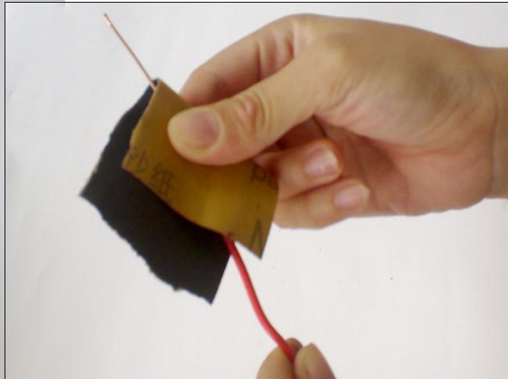
Bước 2 Làm sạch lõi
