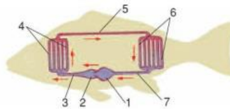
Hình 33.1. Sơ đồ hệ tuần hoàn của cá
